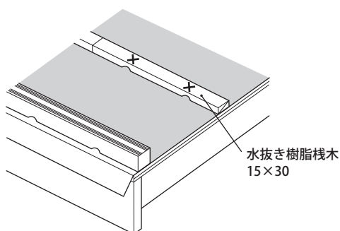
溝が加工された棧木の例
