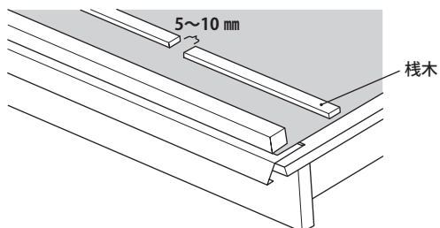
溝が加工された棧木の例
